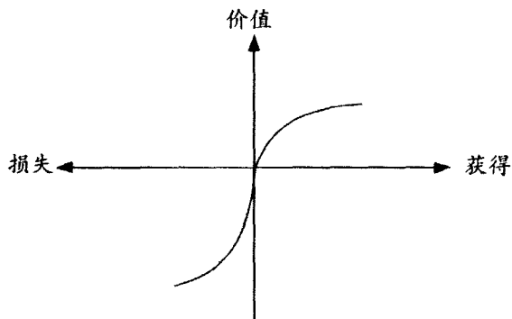
图 13-1 价值函数
